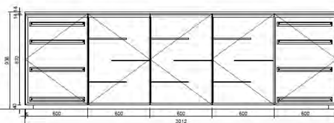
Ansicht Insel aussen
